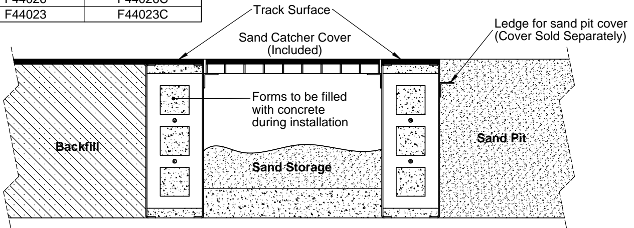
SECTION A-A SCALE 1 : 10
